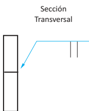
Fig. 65.- Símbolo de la Soldadura Combinada Intermitente y Continua
