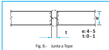
Fig. 8.- Junta a Tope
