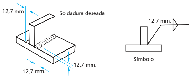
Fig. 72.- Dimensiones de Dos Cordones Iguales de una Soldadura en Ángulo
