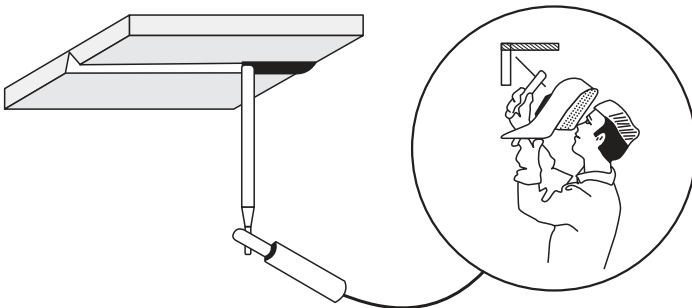
Fig. 5.- Soldadura en Posición Sobrecabeza
