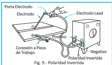
Fig. 9.- Polaridad Invertida
