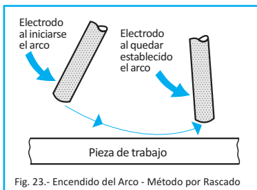
Fig. 23.- Encendido del Arco - Método por Rascado
