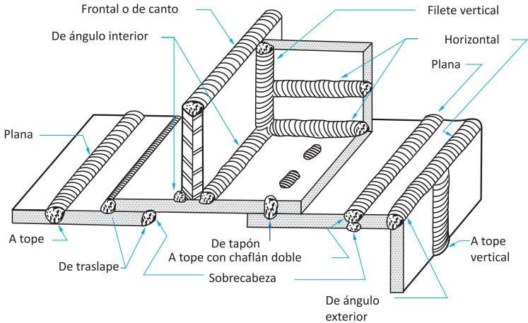
Fig. 1.- Diversas Juntas y Posiciones de Soldadura
