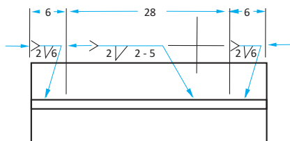
Soldadura deseada
