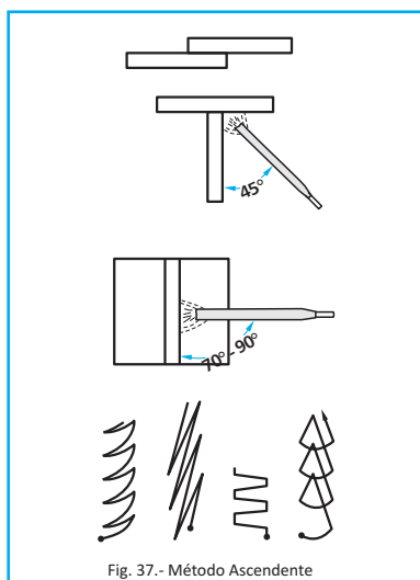
Fig. 37.- Método Ascendente
