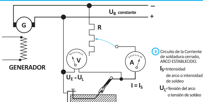
Fig. 14.- Fenómenos de la Soldadura con Transformador
