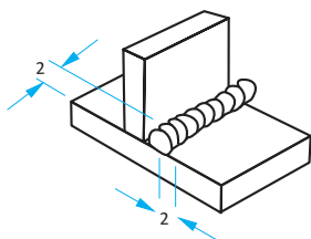
Fig. 71.- Dimensiones de una Soldadura en Ángulo de un solo Cordón
