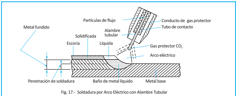
Fig. 17.- Soldadura por Arco Eléctrico con Alambre Tubular
