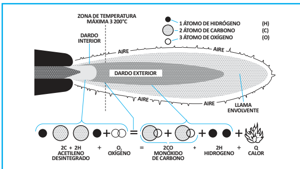
Fig. 24.- Química de la Llama Oxiacetilénica.
