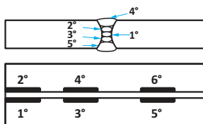
Fig. 55.- Soldadura Alternada
