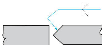
Bisel doble
