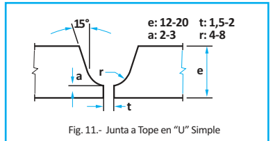
Fig. 11.- Junta a Tope en "U" Simple
