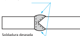
Fig. 79.- Símbolo para el Contorno Convexo de la Cara de Ambos Lados de la Flecha
