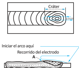
Fig. 25.- Reanudación del Cordón
