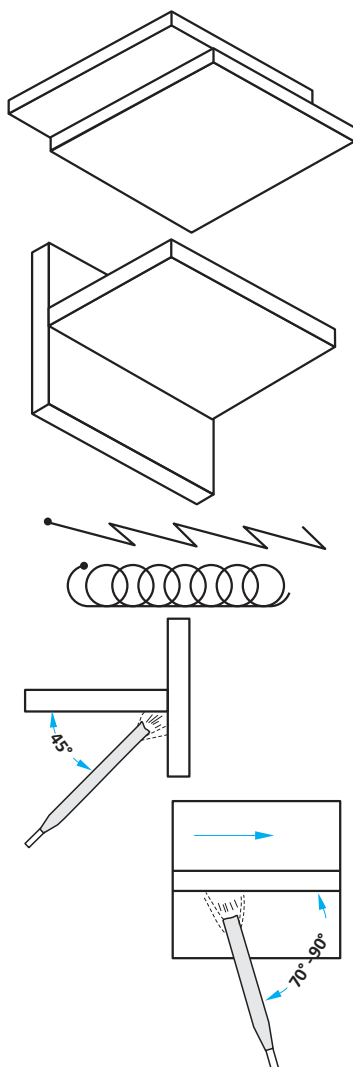
Fig. 40.- Juntas de Traslape y Ángulo
