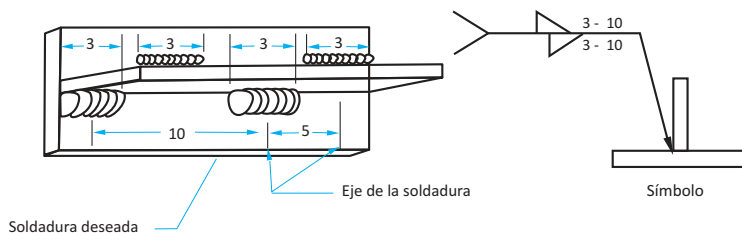
Fig. 64.- Longitud y Separación de las Soldaduras Intermitentes Alternadas
