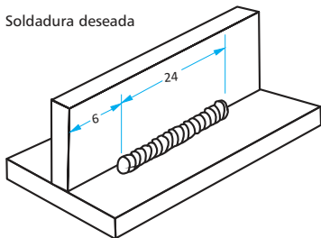
Fig. 70.- Longitud de una Soldadura en Ángulo
