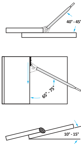
Fig. 32.- Juntas de Solape en Posición Plana
