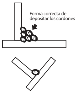
Fig. 31.- Juntas de Ángulo en Posición Plana
