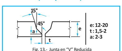
Fig. 13.- Junta en "V" Reducida
