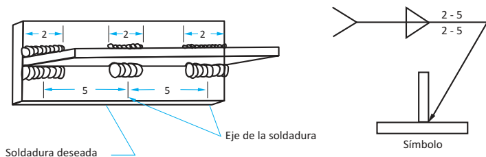
Fig. 63.- Longitud y Separación de las Soldaduras Intermitentes Opuestas
