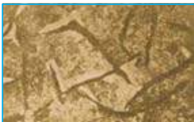
Fig. 3.- Fundición Gris Perlítica
