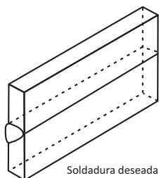
Fig. 67.- Símbolo de la Soldadura a Tope sin Chaflán del Lado Opuesto a la Flecha
