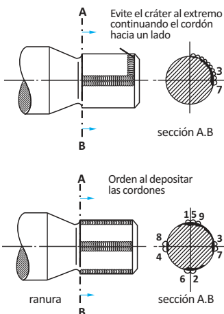
Fig. 30.- Rellenado de un Eje
