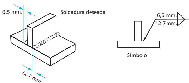
Fig. 73.- Dimensiones del Cordón de Lados Desiguales en una Soldadura en Ángulo
