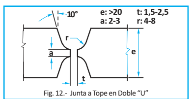
Fig. 12.- Junta a Tope en Doble "U"
