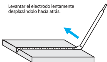
Fig. 26.- Relleno de Cráter
