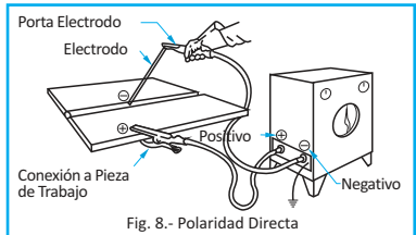
Fig. 8.- Polaridad Directa
