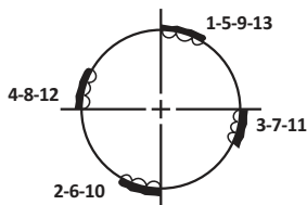
Fig. 56.- Soldadura de Ejes
