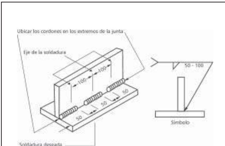
Fig. 62.- Longitud y Separación de las Soldaduras Intermitentes
