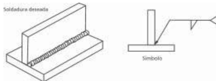
Fig. 69.- Soldadura en Angulo Continuo
