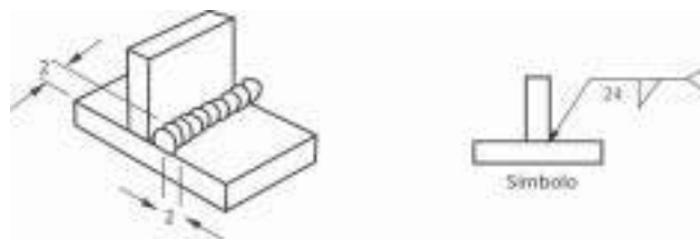
Fig. 71.- Dimensiones de una Soldadura en Angulo de un solo Cordón
