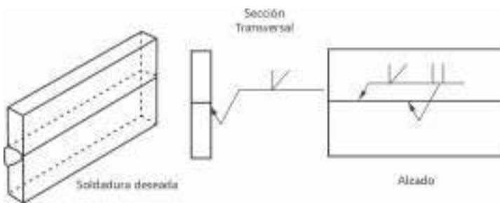
Fig. 76.- Símbolo de la Soldadura a Tope sin Chafán del Lado Opuesto a la Flecha
