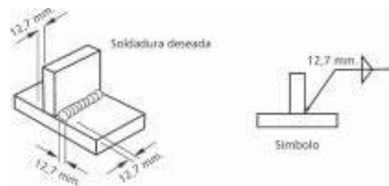
Fig. 72.- Dimensiones de Dos Cordones Iguales de una Soldadura en Angulo
