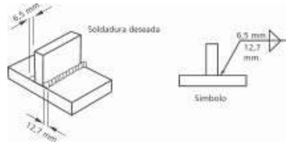
Fig. 73.- Dimensiones del Cordón de Lados Desiguales en una Soldadura en Angulo
