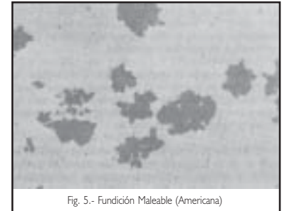
Fig. 5.- Fundición Maleable (Americana)
