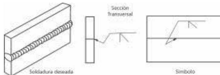
Fig. 75.- Símbolo de la Soldadura a Tope con Chaflán en el Lado Próximo a la Flecha
