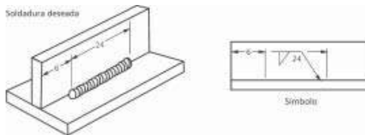
Fig. 70.- Longitud de una Soldadura en Angulo
