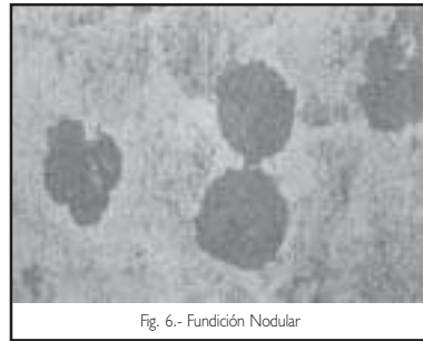
Fig. 6.- Fundición Nodular
