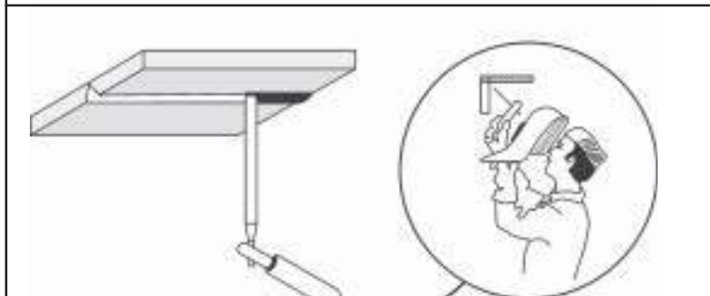
Fig. 4.- Soldadura en Posición Horizontal
