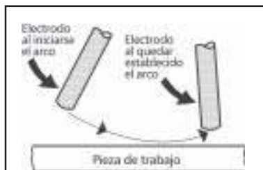
Fig. 23.- Encendido del Arco - Método por Rascado
