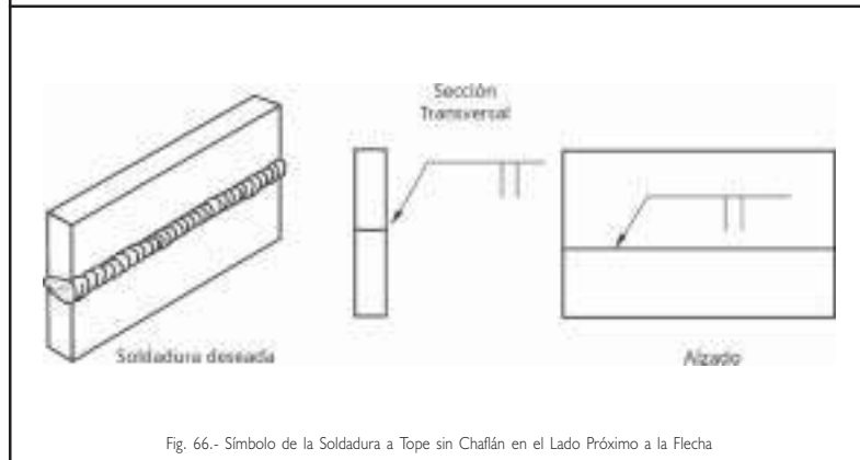
Fig. 66.- Símbolo de la Soldadura a Tope sin Chafán en el Lado Próximo a la Flecha
