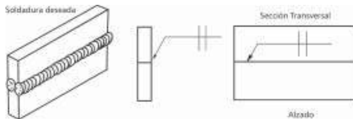
Fig. 68.- Símbolo de la Soldadura a Tope sin Chafán de Ambos Lados de la Flecha
