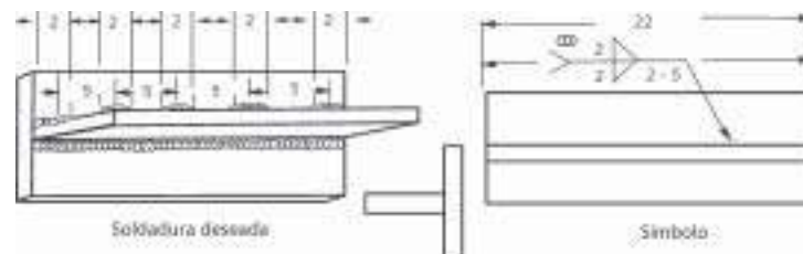
Fig. 74.- Soldadura Combinada Intermitente y Continua (Lados Opuestos de Junta)
