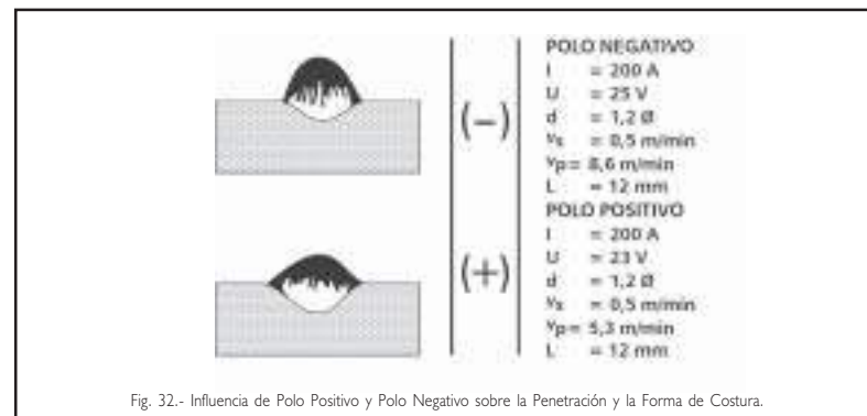
Fig. 32.- Influencia de Polo Positivo y Polo Negativo sobre la Penetración y la Forma de Costura.
